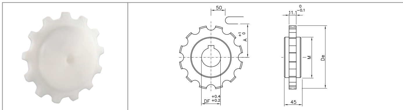
Standard sprockets material: polyamide
